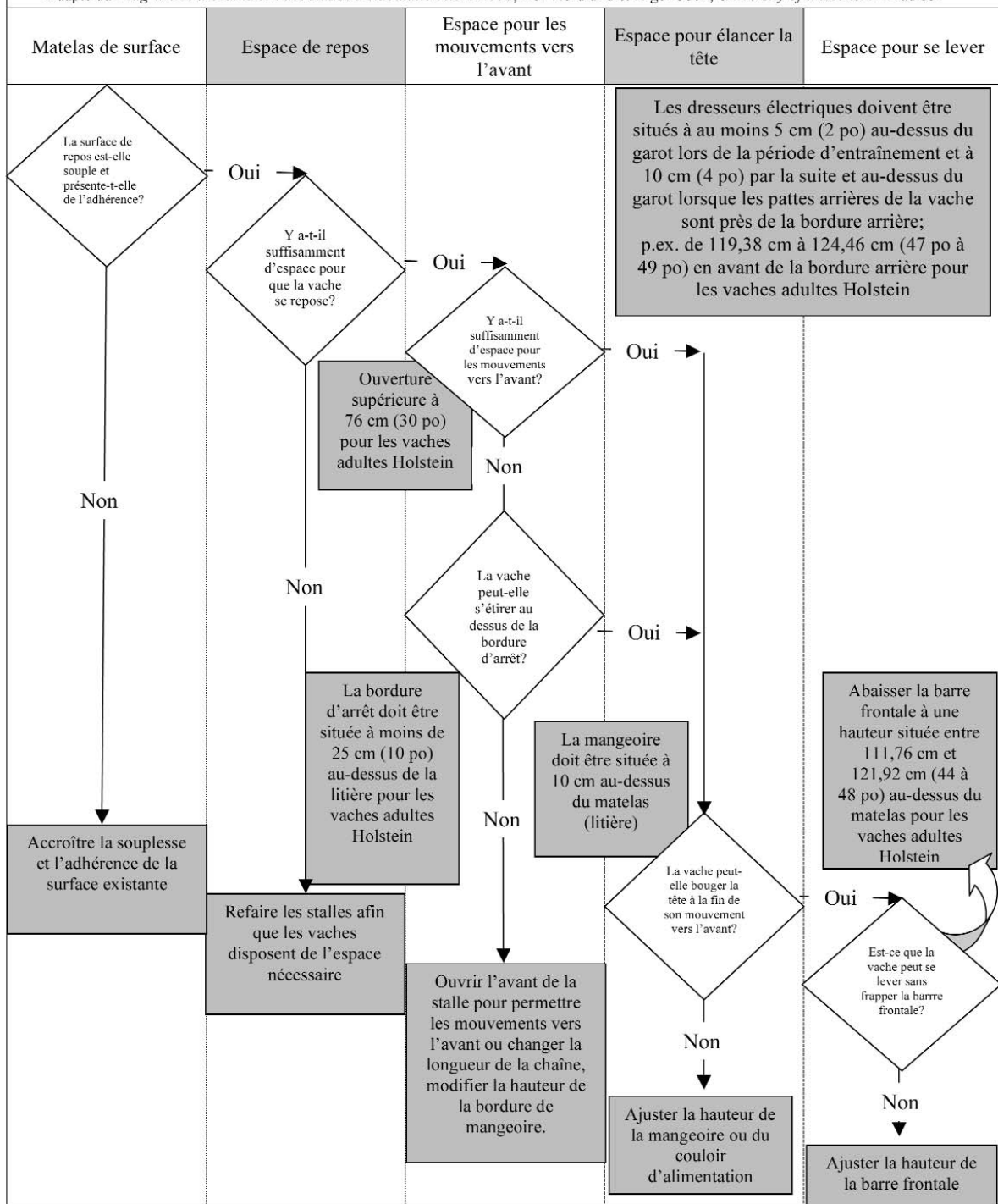
Diagramme d'évaluation des stalles à stabulation entravée 2008v2
